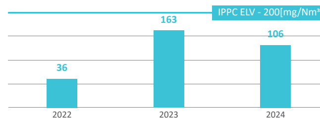
Figura 2 Emëtimet SOx
